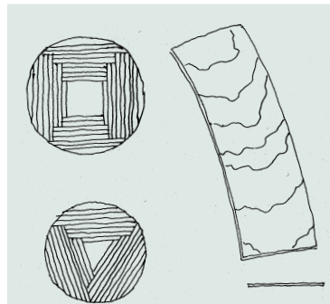
Hyvlat stickspån. Träets fibrer är delvis avskurna, spånen blir böjliga och utsidan har fjäll. Fjällen skall peka ut och ned över taket. Då rinner vattnet bort från veden. Om spånen läggs fel samlas regnvatten i fickorna.
