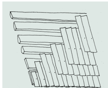
Trelagstäckning. Börja nerifrån. Första lagret används 1/3 spån, nästa 2/3 och tredje lagret ett helt spån.
