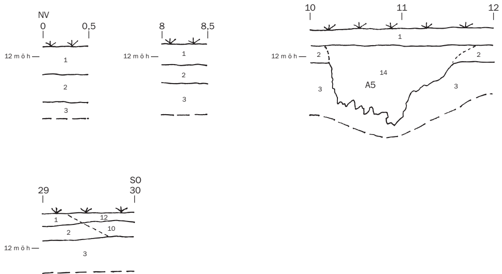
Sektion 6, schakt 6. Skala 1:40.
