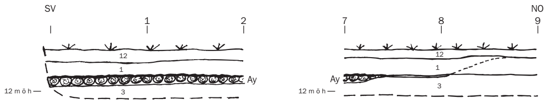
Sektion 5, schakt 5. Skala 1:40.
