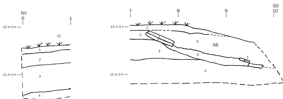
Sektion 1, schakt 1. Skala 1:40.
