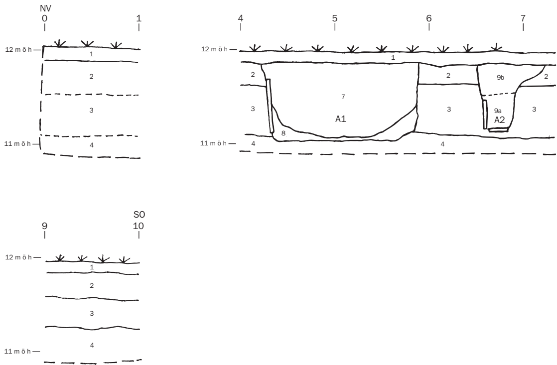
Sektion 2, schakt 2. Skala 1:40.
