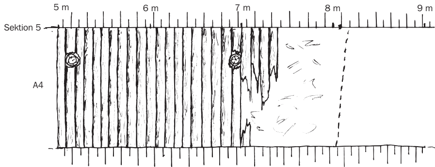
Plan över anläggning 4 i sektion 5. Skala 1:40.
