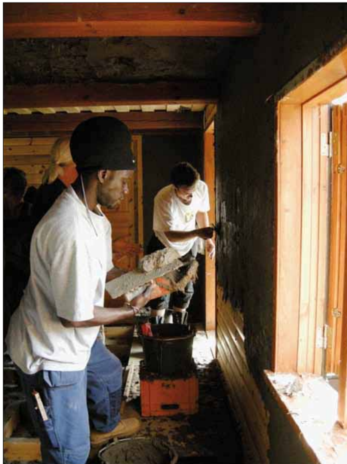
Deltagarna inom Byggnadsvård & Sysselsättning utövar lerklining.
