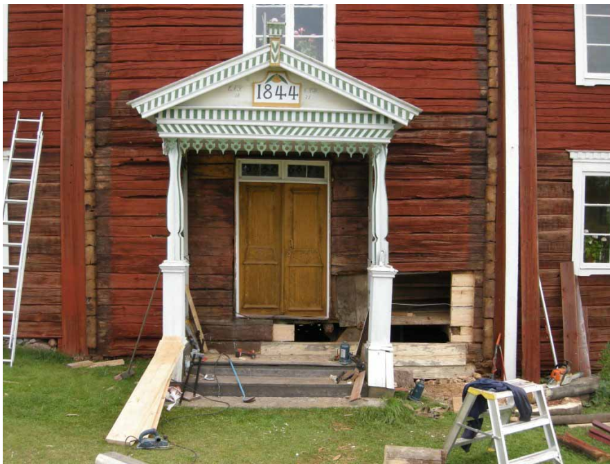
Ill. 12. Brokvisten under renoveringen med rötskadade stockar i mangårdsbyggnadens nordvästra fasad borttagna. Foto från nordväst: Daniel Olsson, Läns museet Gävleborg 2009-08-25.
