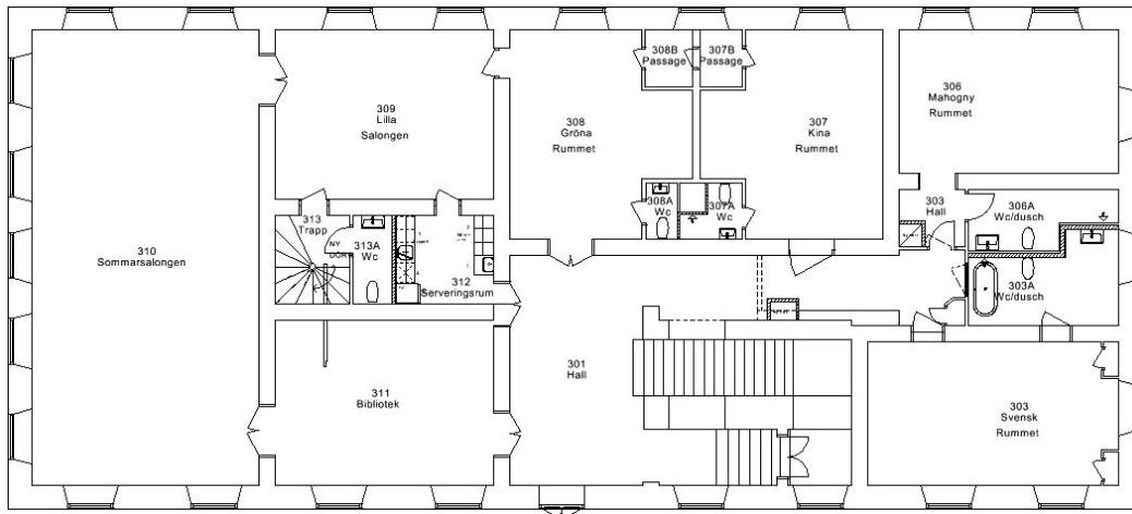
Bild 40. Den planlösning som herrgården får i samband med 2014 års ombyggnation. Ritning Marcus Olhans, Arkitektgruppen GKAK.
