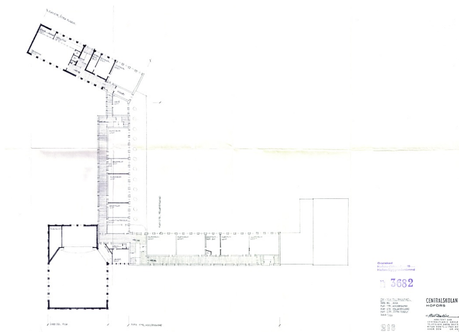
Planritning över Hagaskolans första plan, med nytillkomna delar 1968. Ritningen är signerad Sten Dalén och daterad 1964. Högst upp syns slöjdsalsdelen i två hela våningar. Auladelen och gymnastikdelen har två plan. Ritningarna förvaras på Kommunarkivet i Hofors.
