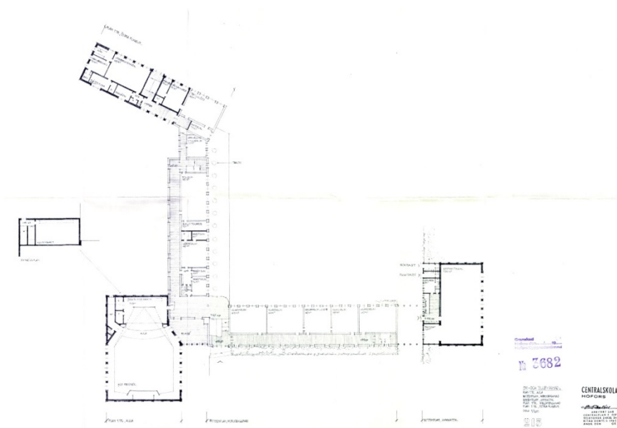
Planritning över Hagaskolans första plan, med nytillkomna delar 1968. Ritningen är signerad Sten Dalén och daterad 1964. Högst upp syns slöjdsalsdelen som dockades mot specialrumsflygelns östra gavel. Mellan de ursprungliga flyglarna, i det nordvästra hörnet, tillkom auladelen som på första våningen rymde just aula. Mot söder syns gymnastiksalen. Ritningarna förvaras på Kommunarkivet i Hofors.
