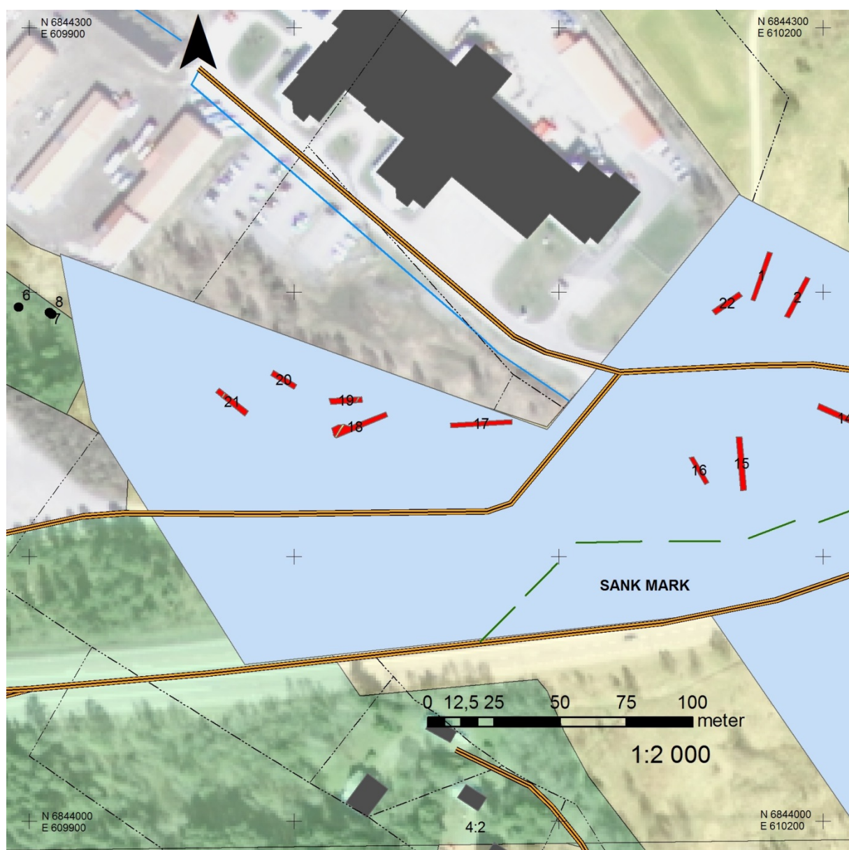
Figur 5. Utredningsområdets västra del med sökschakten rödmarkerade, se bilaga 1. Svarta markeringar visar nyfunna lämningar direkt utanför områdets begränsning i väster, se bilaga 3.
