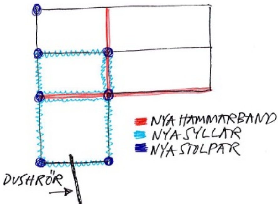
Figur 7. Skissen visar bytta syllar, stolpar och hammarband. Skiss: Ulrika Olsson, Läns museet Gävleborg, 2018-09-27.
