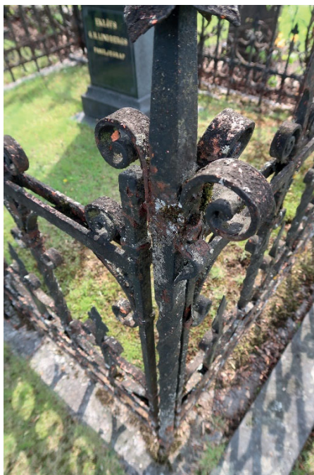
Figur 7–9. K7:0027 med staket i smide, innan påbörjade arbeten. Staketet uppvisade kraftiga rostangrepp och lösa delar. Foto: Ulrika Olsson, Läns museet Gävleborg, 2019-05-20.
