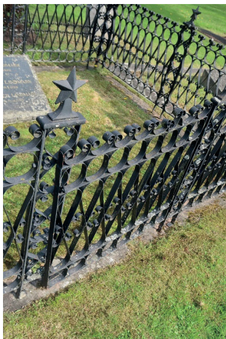
Figur 41–43. K7:0190 med staket i smide, innan påbörjade arbeten. Staketet uppvisade kraftiga rostangrepp och biologisk påväxt. Foto: Ulrika Olsson, Läns museet Gävleborg, 2019-05-20.
