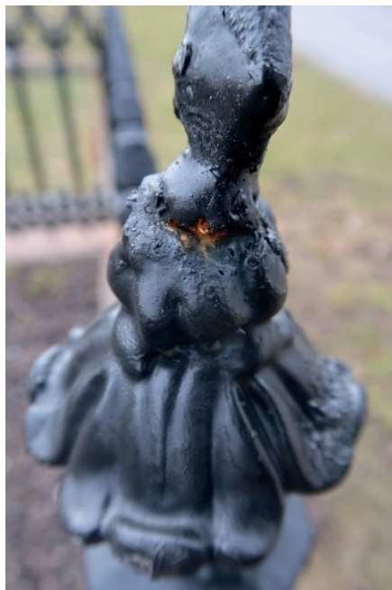
Figur 24–26. K7:0125 med staket i gjutjärn, efter avslutade arbeten. Här syns några missar i målningsarbetet, samt skador tillkomna på grund av att färgen förmodligen inte torkar riktigt innan återmontering. Möjligen är färgen påförd för tjockt med följd att endast det yttersta lagret torkat men inte de underliggande. Foto: Ulrika Olsson, Läns museet Gävleborg, 2020-03-18.
