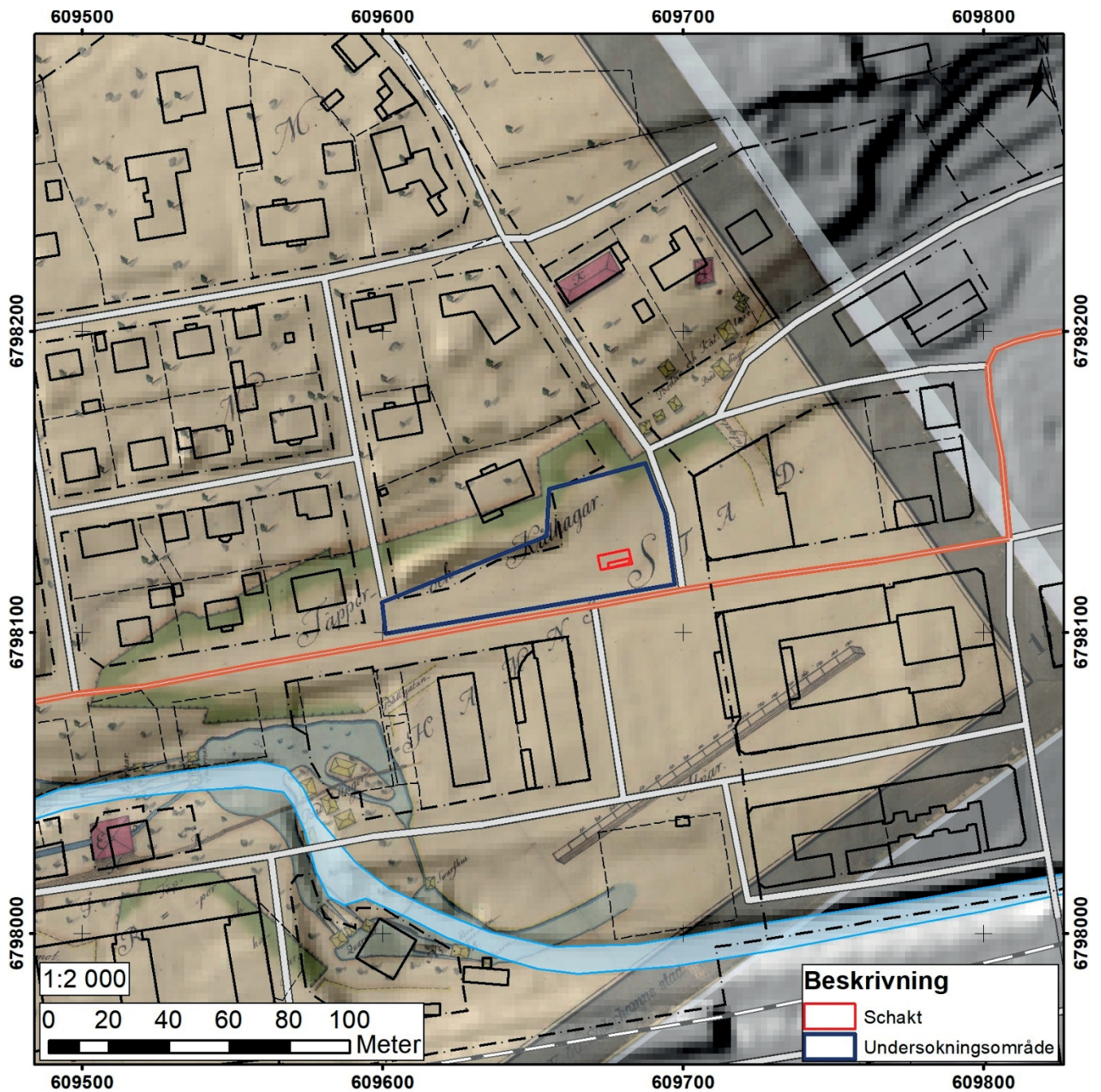
Figur 6. Utdrag ur Lantmäteriets fastighetskarta. I bakgrunden ligger en avmätningsskarta över Söderhamns stad år 1749 (LMS V50-1:4). Skala 1:2 000.
