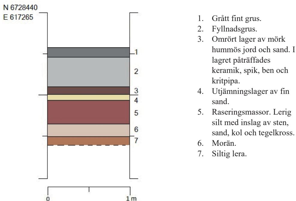
Figur 8. Profilritning av lagerföljden i det undersökta schaktet. Sektionens position redovisas i figur 7.
