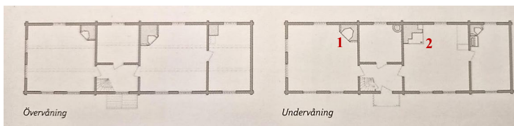
Figur 6. Gäststugubyggningens planlösning med spisen i herrstugan markerad med nummer 1 och spisen i mellanstugan markerad som nummer 2. Planritning ur skriften Världsarvsgården Kristofers.
